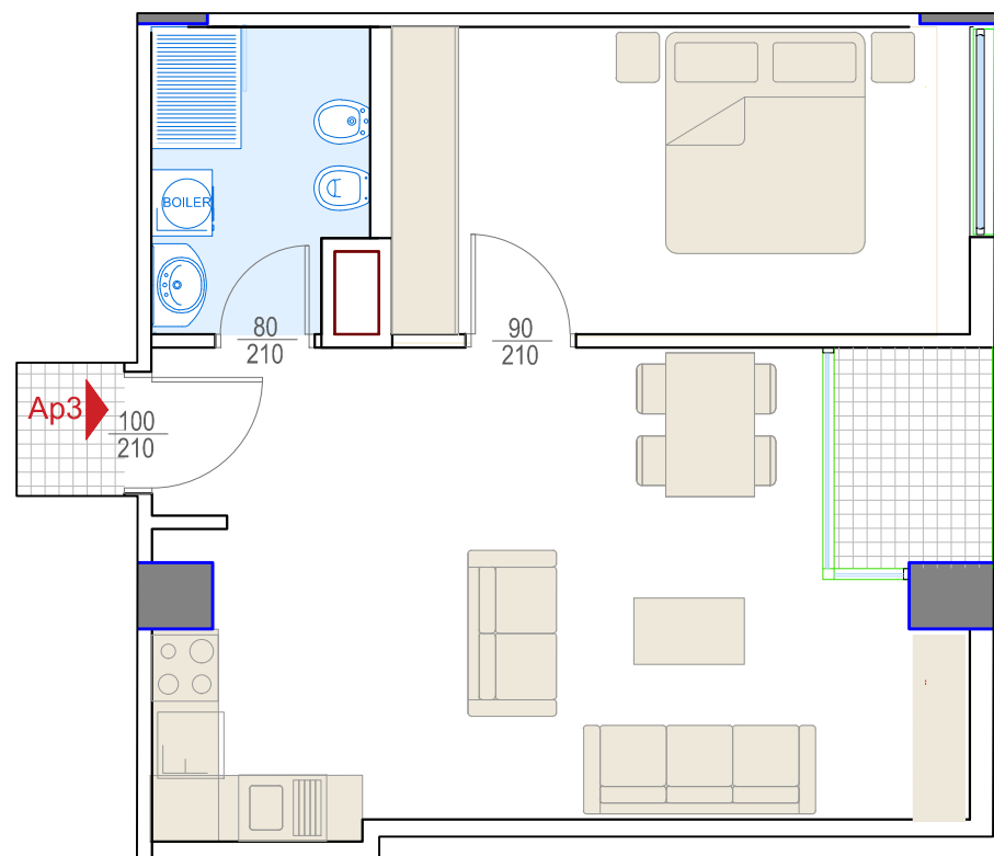
Planimetri Sh. 1:75 - Mobilimi -
