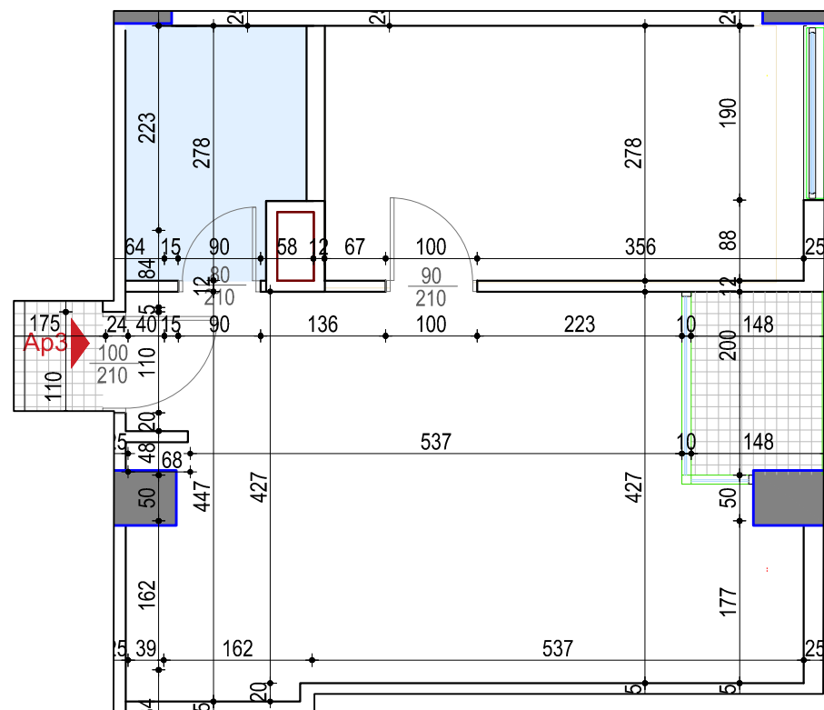
Planimetri Sh. 1:75 - Dimensionimi -
