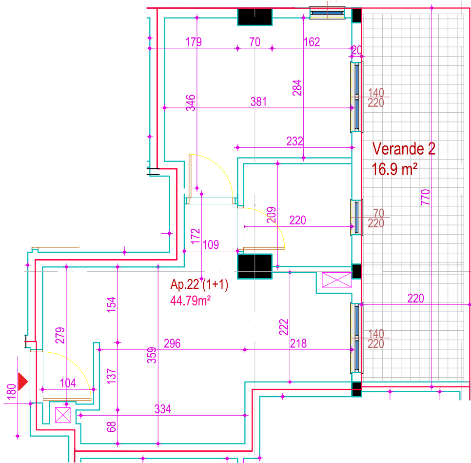
Planimetri Sh. 1:75 - Dimensionimi -
