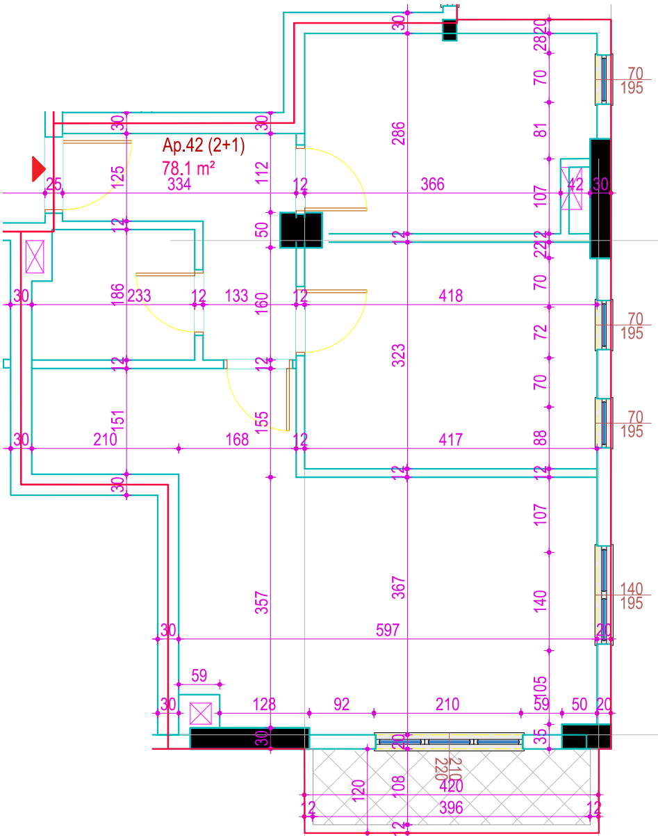
Pozicioni i apartamentit ne planin e objektit
