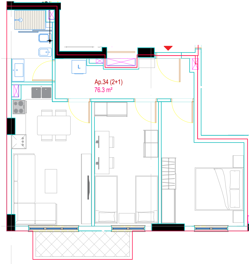
Planimetri Sh. 1:75 - Mobilimi -
