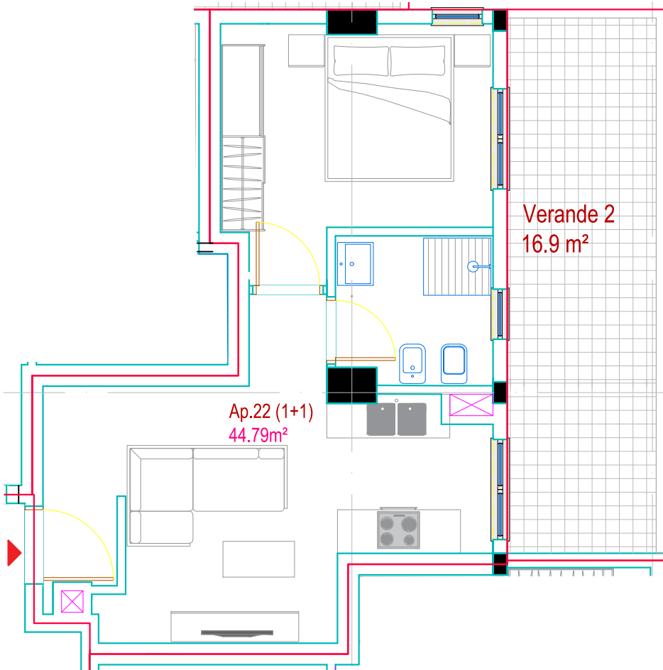
Planimetri Sh. 1:75 - Mobilimi -
