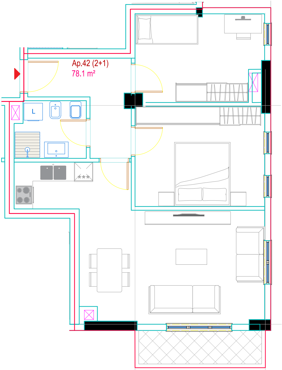
Planimetri Sh. 1:75 - Mobilimi -
