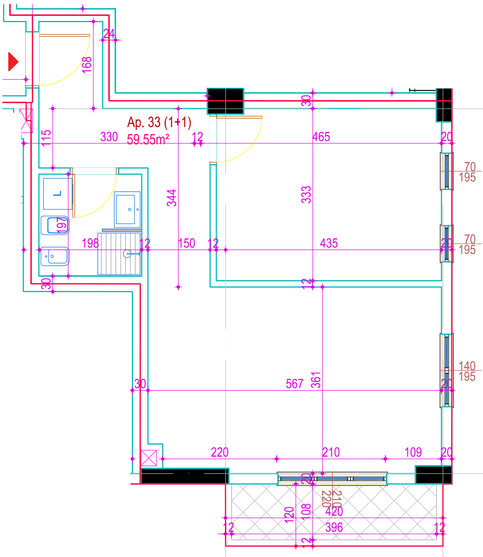
Pozicioni i apartamentit ne planin e objektit
