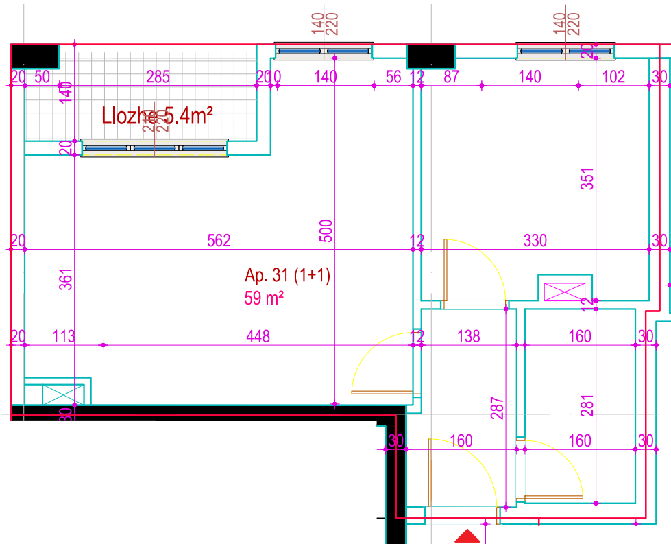
Planimetri Sh. 1:75 - Dimensionimi -
