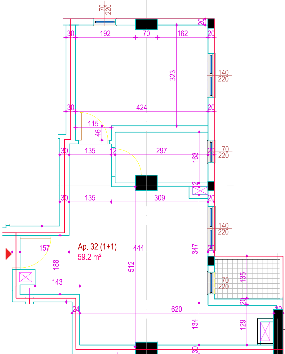
Planimetri Sh. 1:75 - Dimensionimi -
