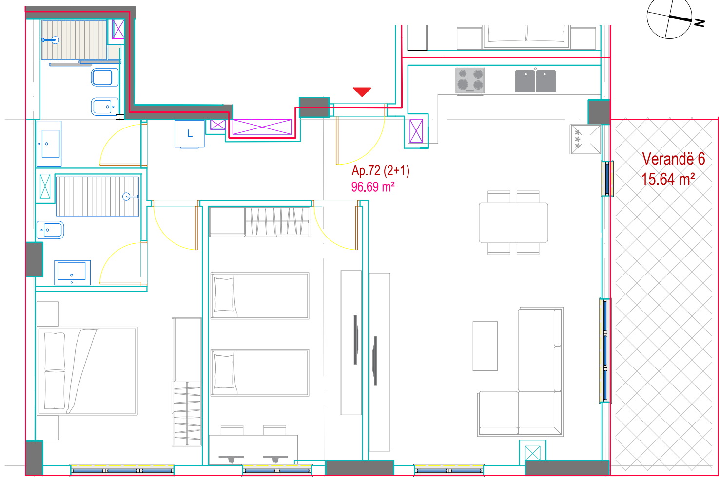
Planimetri Sh. 1:75 - Mobilimi -
