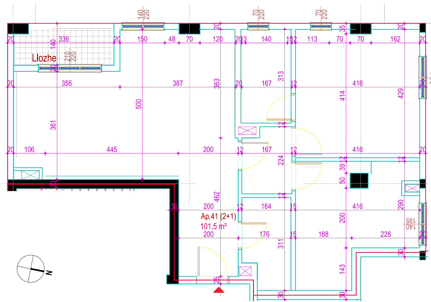
Planimetri Sh. 1:75 - Dimensionimi -
