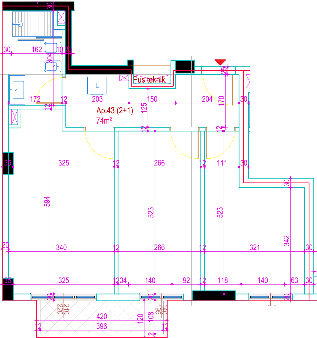
Pozicioni i apartamentit ne planin e objektit
