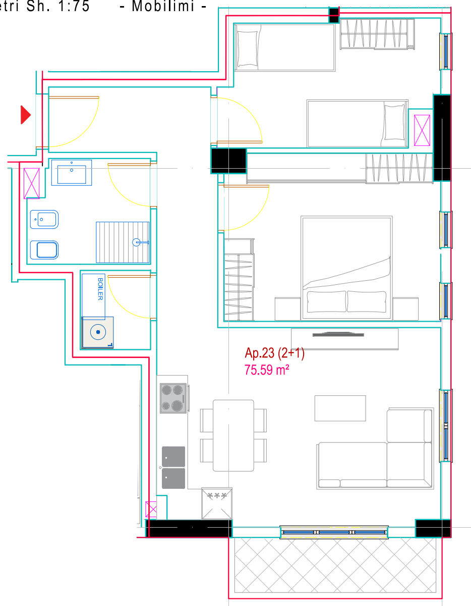
Planimetri Sh. 1:75 - Mobilimi -
