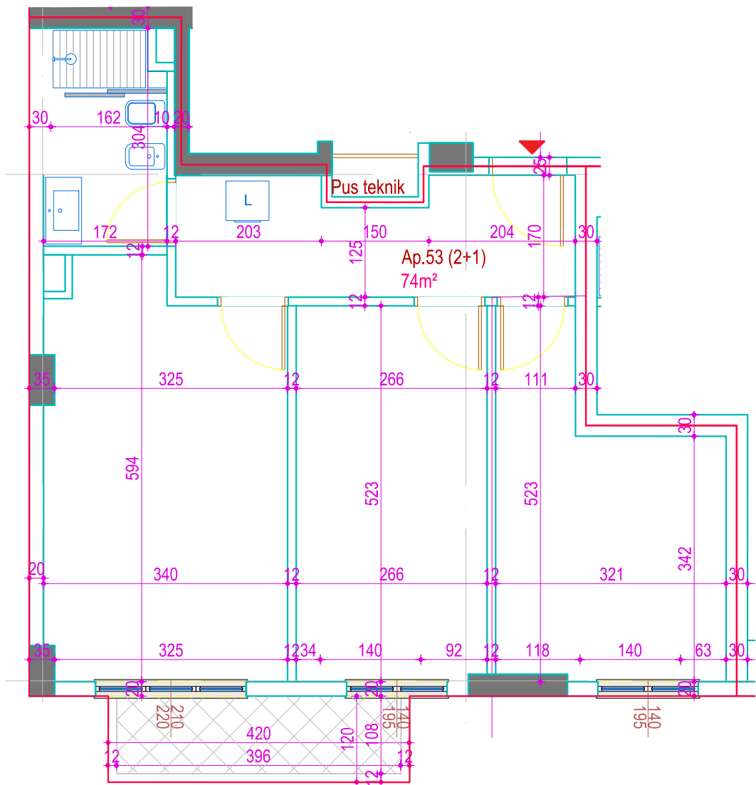
Pozicioni i apartamentit ne planin e objektit
