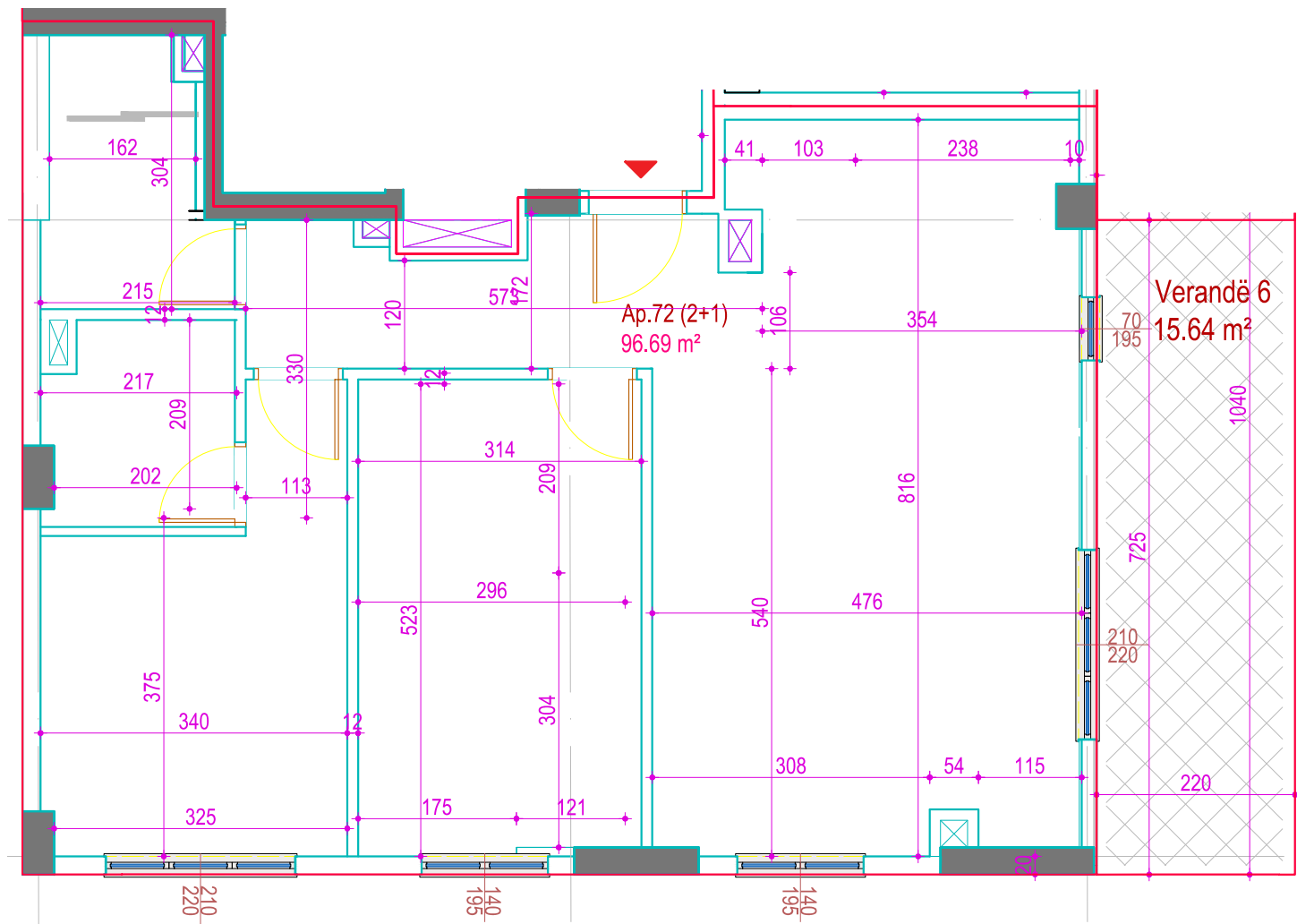
Planimetri Sh. 1:75 - Dimensionimi -
