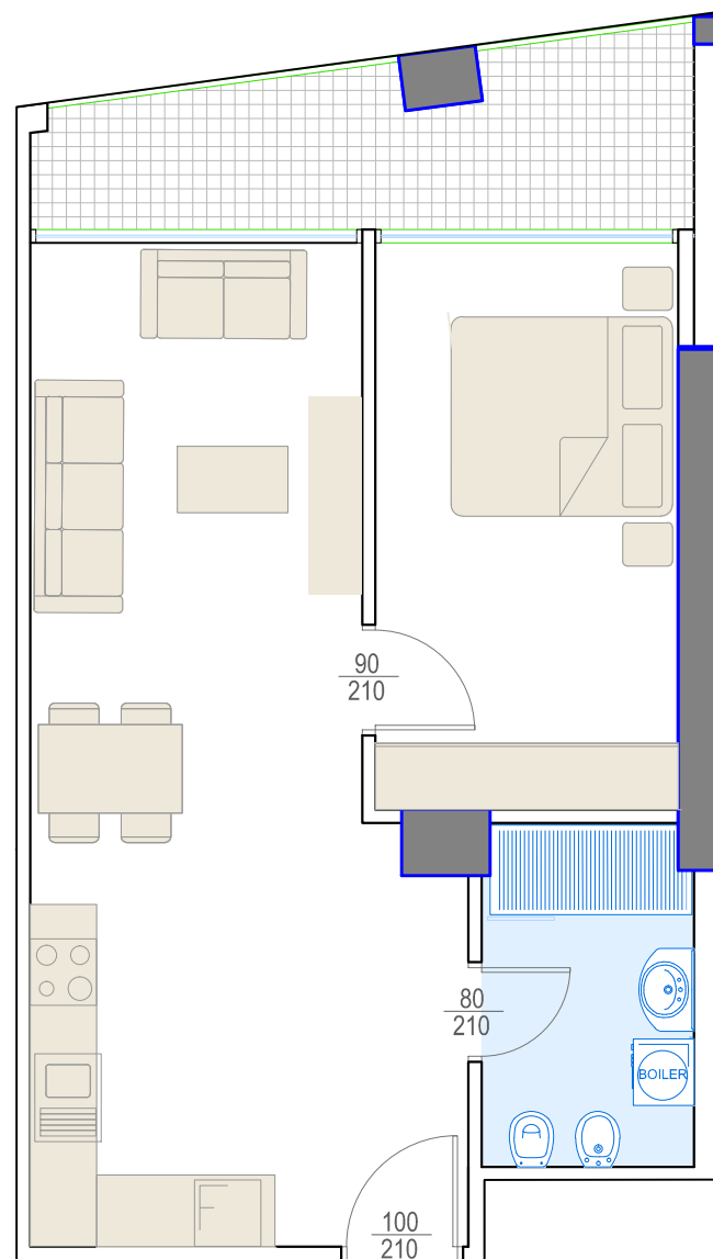
Planimetri Sh. 1:75 - Mobilimi -
