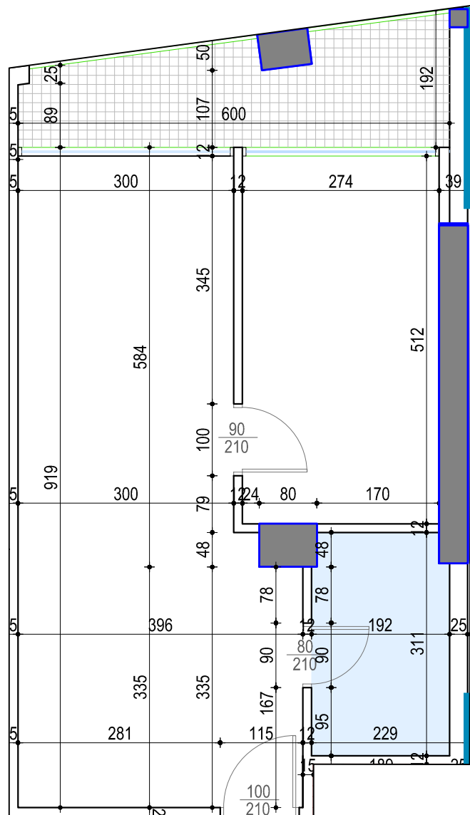
Planimetri Sh. 1:75 - Dimensionimi -
